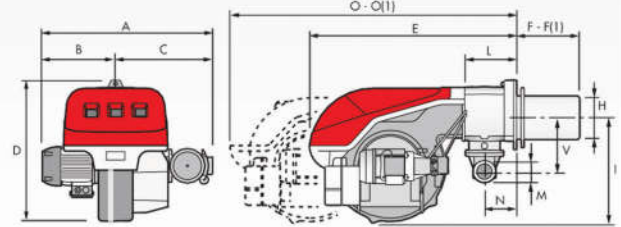
GRLS 70 - 100 - 130 - 190 - 250
